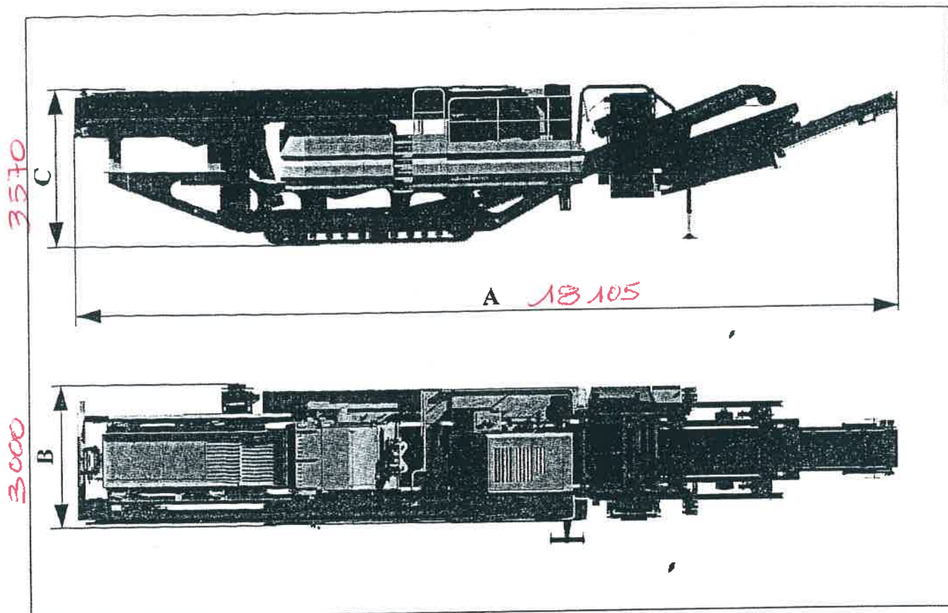
Figure 3-4 Unité LT1213S en position de transport
